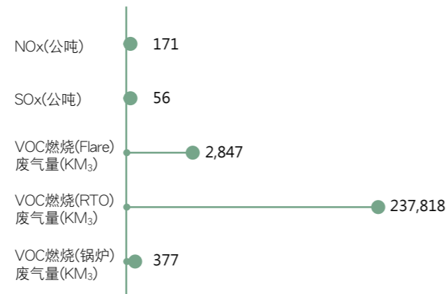
2018 年台橡集团各类空污排放量
