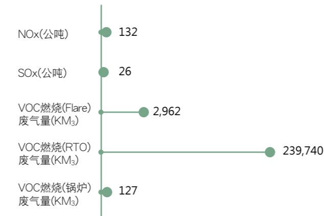
2019 年台橡集团各类空污排放量
